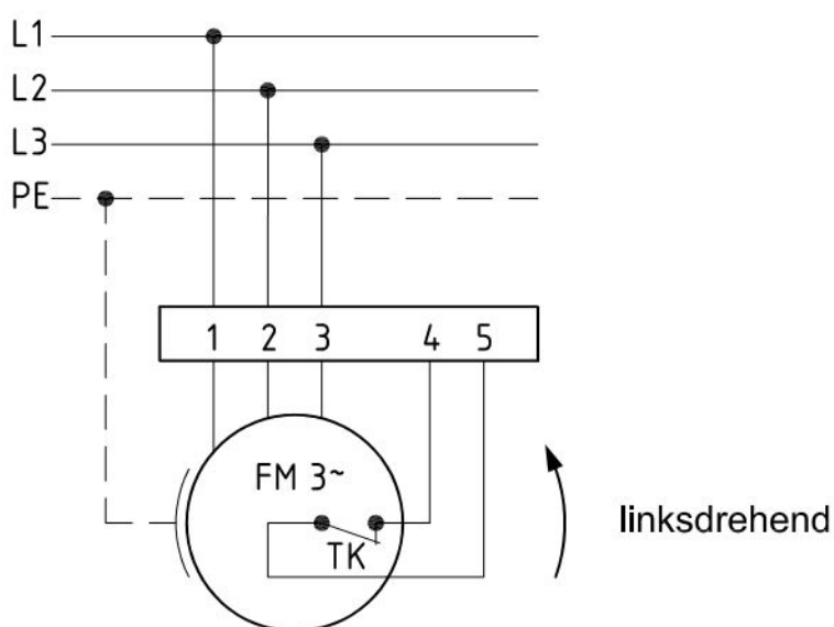
Anschlußplan 0.13-2 l.
