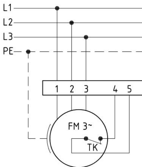
Anschlußplan 0.13-2 I.
