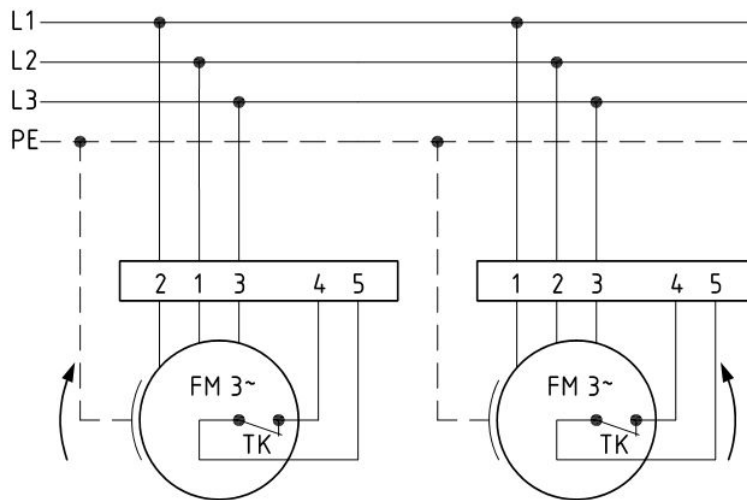
Anschlußplan 0.16-1 / 0.16a-1
