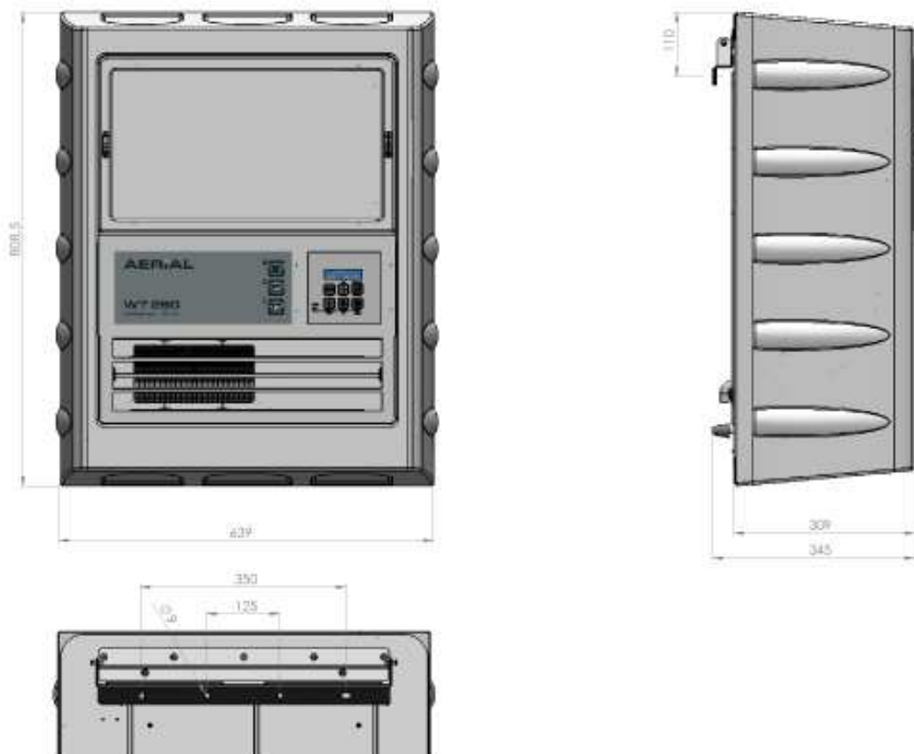
Abb. 2: Maßzeichnung
