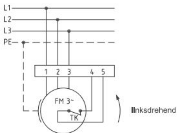
Anschlußplan 0.13-2 I.
