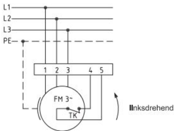
Anschlußplan 0.13-2 I.
