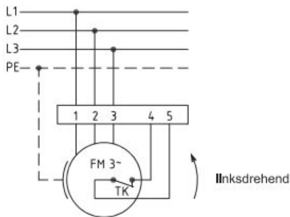
Anschlußplan 0.13-2 I.
