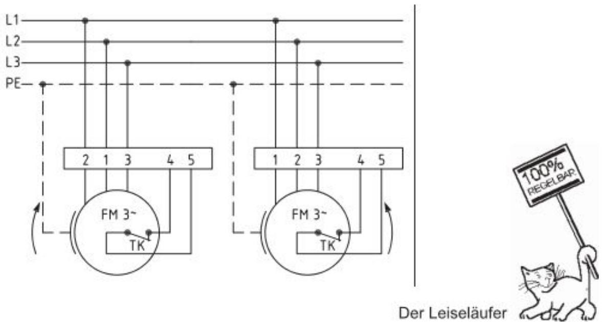
Anschlußplan 0.16-1 / 0.16a-1
