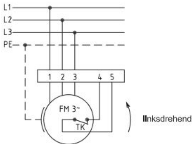
Anschlußplan 0.13-2 I.
