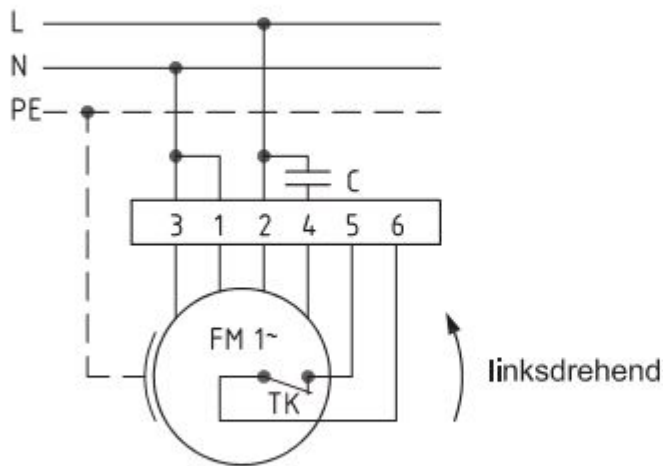
Anschlußplan 0.11-1 I
