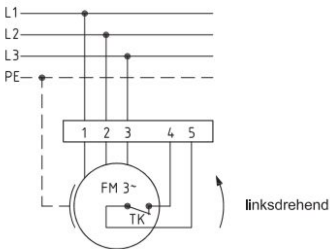
Anschlußplan 0.13-2 I
