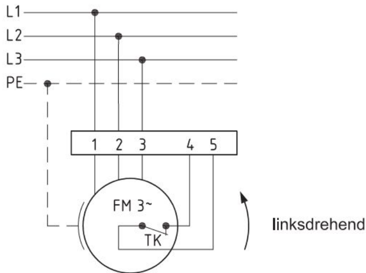
Anschlußplan 0.13-2 I
