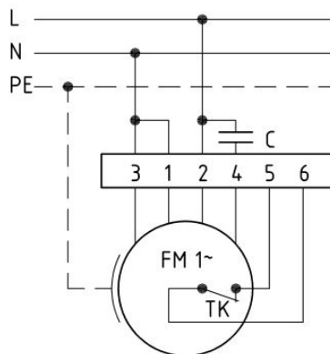
Anschlußplan 0.11-1 l.
