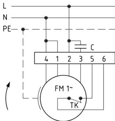
Anschlußplan 0.11-1 r.
