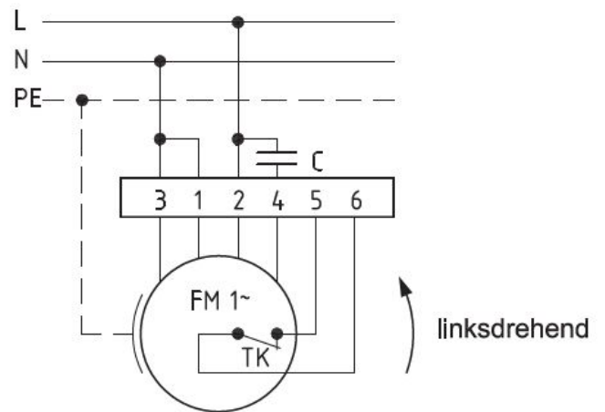
Anschlußplan 0.11-1 l.
