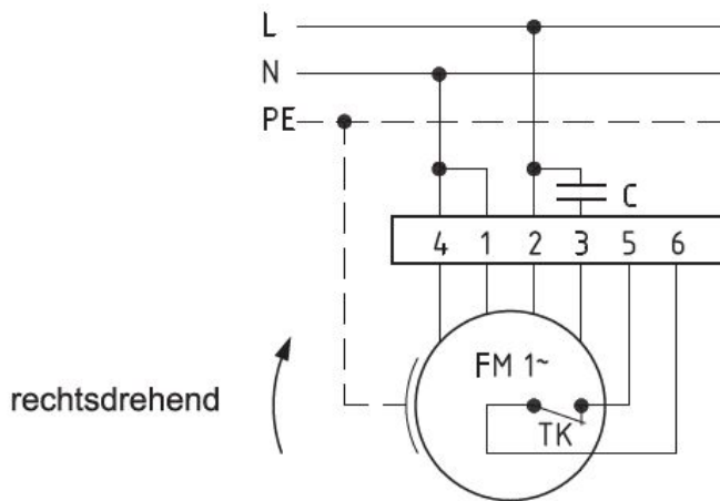
Anschlußplan 0.11-1 r.
