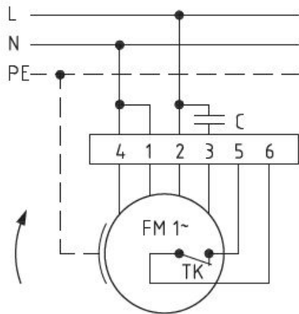
Anschlußplan 0.11-1 r.
