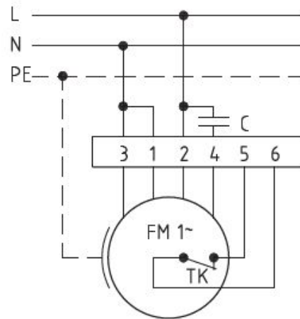
Anschlußplan 0.11-1 l.
