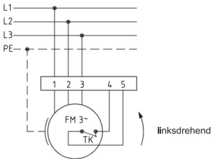
Anschlußplan 0.13-2 I.
