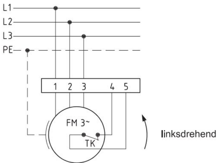
Anschlußplan 0.13-2 I.
