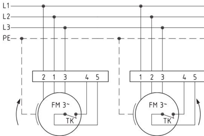
Anschlußplan 0.16-1 / 0.16a-1
