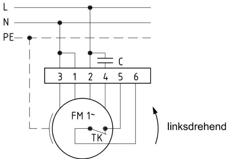
Anschlußplan 0.11-1 I.
