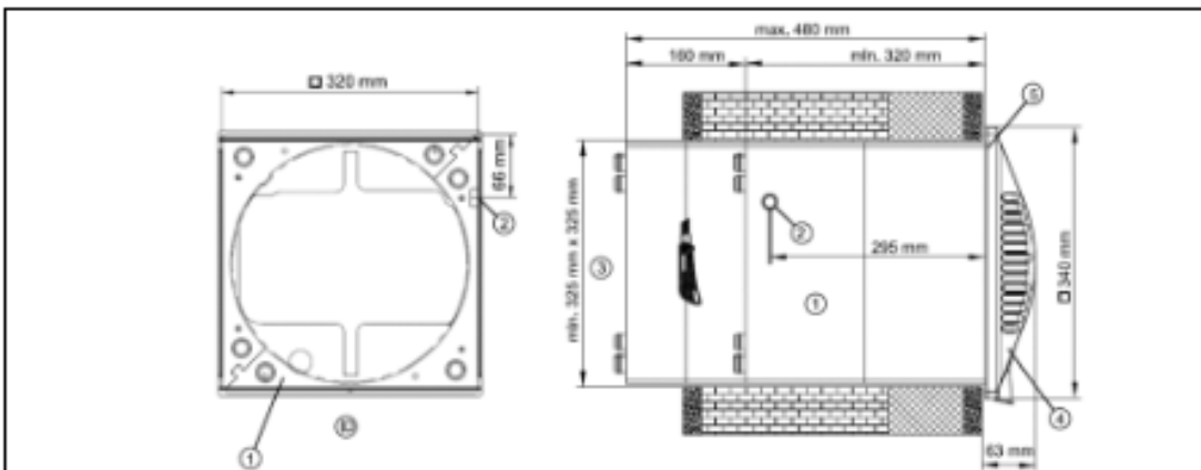
Abb. 3.3 Einbaumaße quadratische Wandhülse
