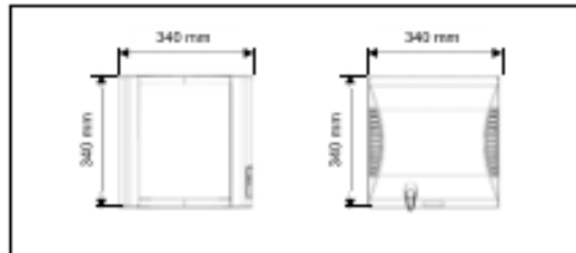
Abb. 3.2 Abmaße Innenblende und Außenblende
