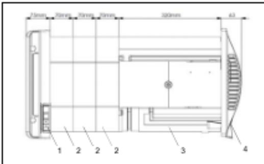
Abb. 3.1 Abmaße Lüftungsgerät
