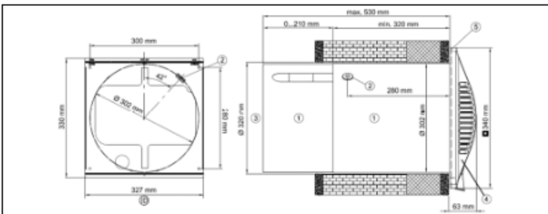
Abb. 3.4 Einbaumaße runde Wandhülse
