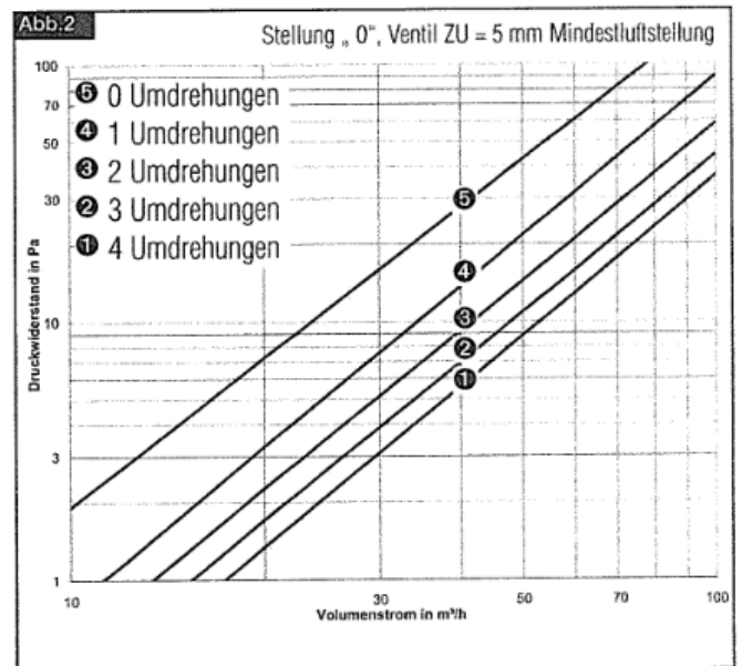
4.0 Kennlinie DLV 100: Zuluft ohne Filter
