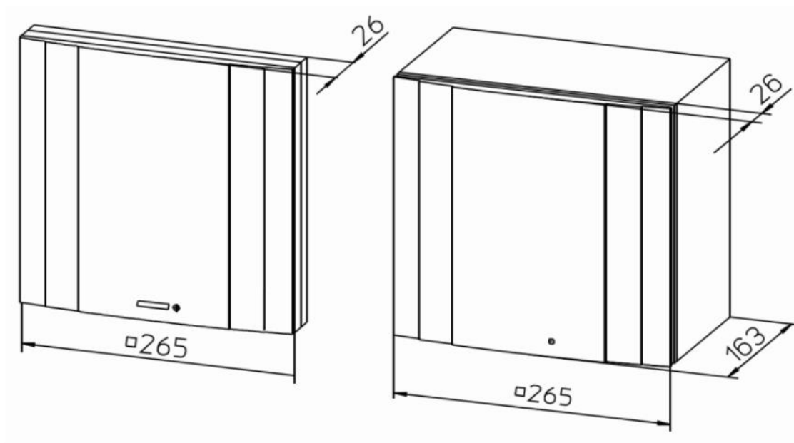
Masse / Dimensions / Dimensioni, mm
