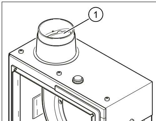
Abb. 5: Funktion der Rückschlagklappe überprüfen
