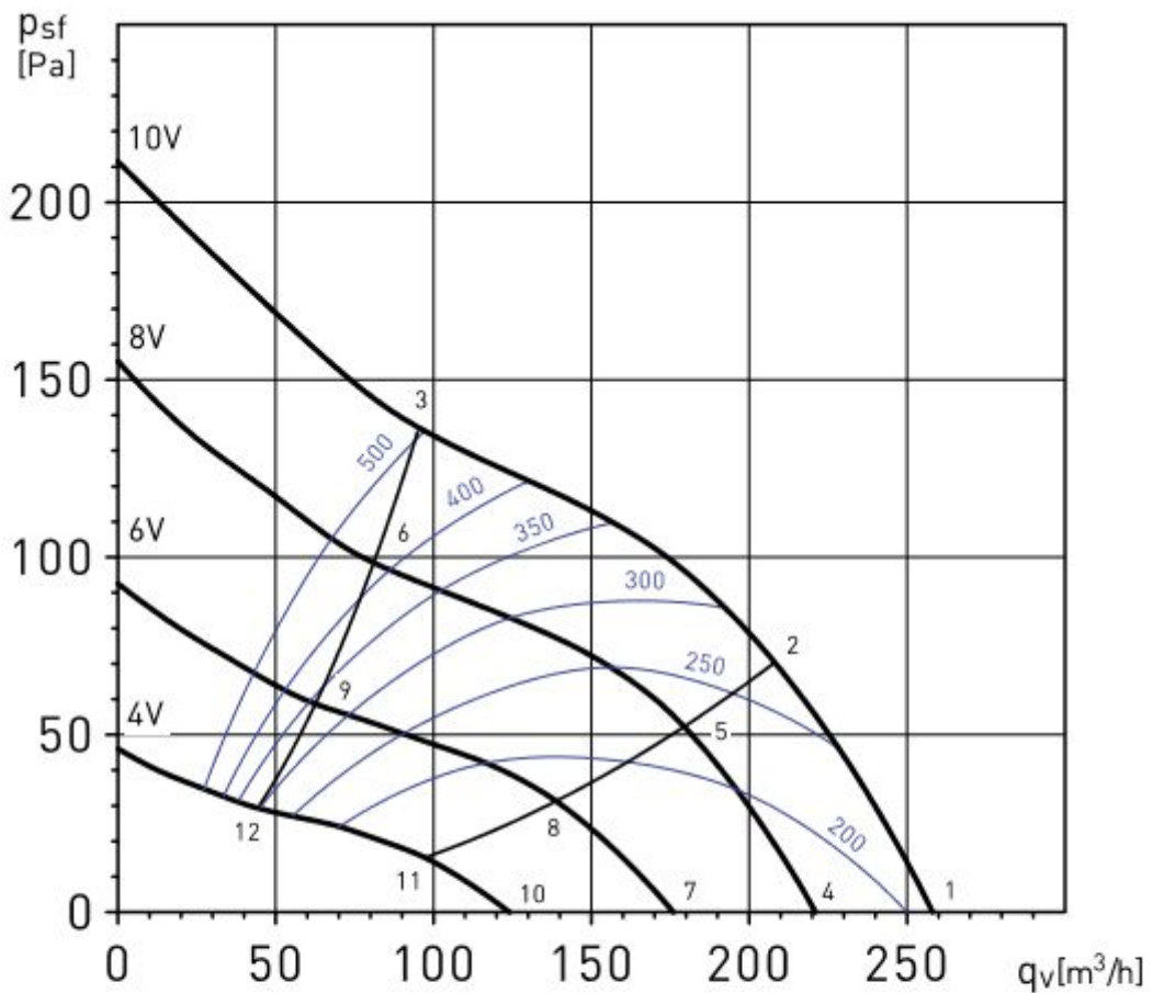
JETLINE-100 ECOWATT
