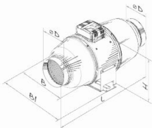
Iso-Mix 100 – Iso-Mix 150
