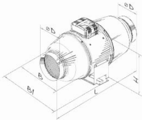
Iso-Mix 100 – Iso-Mix 150
