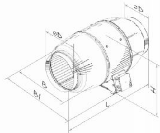
Iso-Mix 160 – Iso-Mix 315
