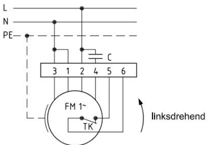
Anschlußplan 0.11-1 I.
