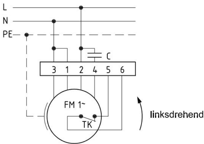
Anschlußplan 0.11-1 I.
