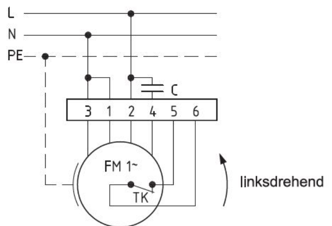
Anschlußplan 0.11-1 l.
