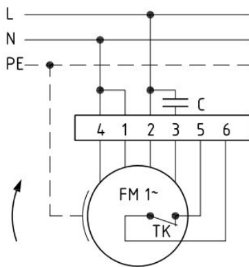
Anschlußplan 0.11-1 r.
