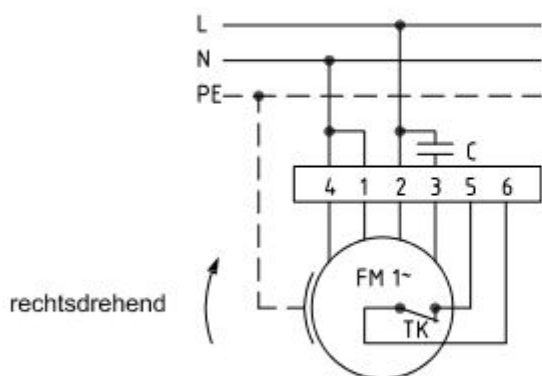
Anschlußplan 0.11-1 r.
