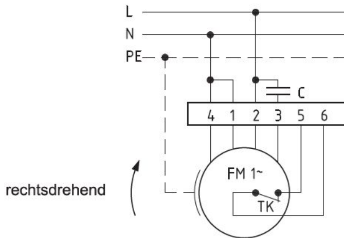
Anschlußplan 0.11-1 r.
