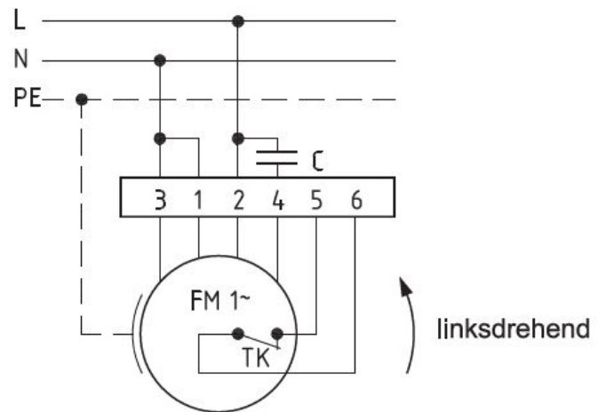
Anschlußplan 0.11-1 l.
