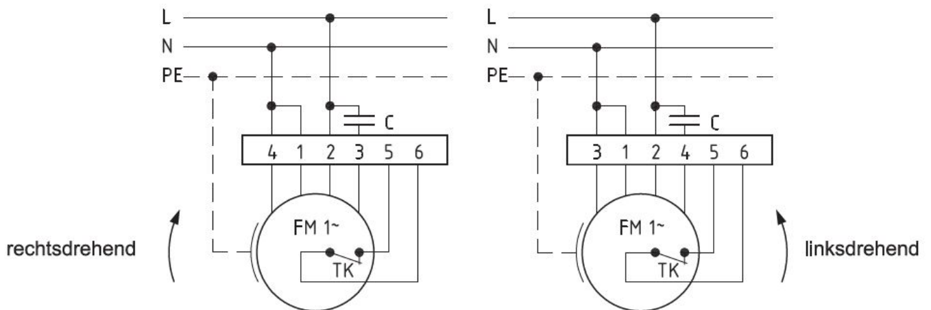
Anschlußplan 0.11-1 r.
