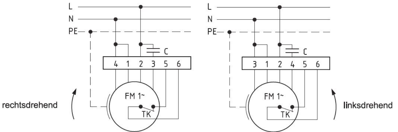
Anschlußplan 0.11-1 r.
