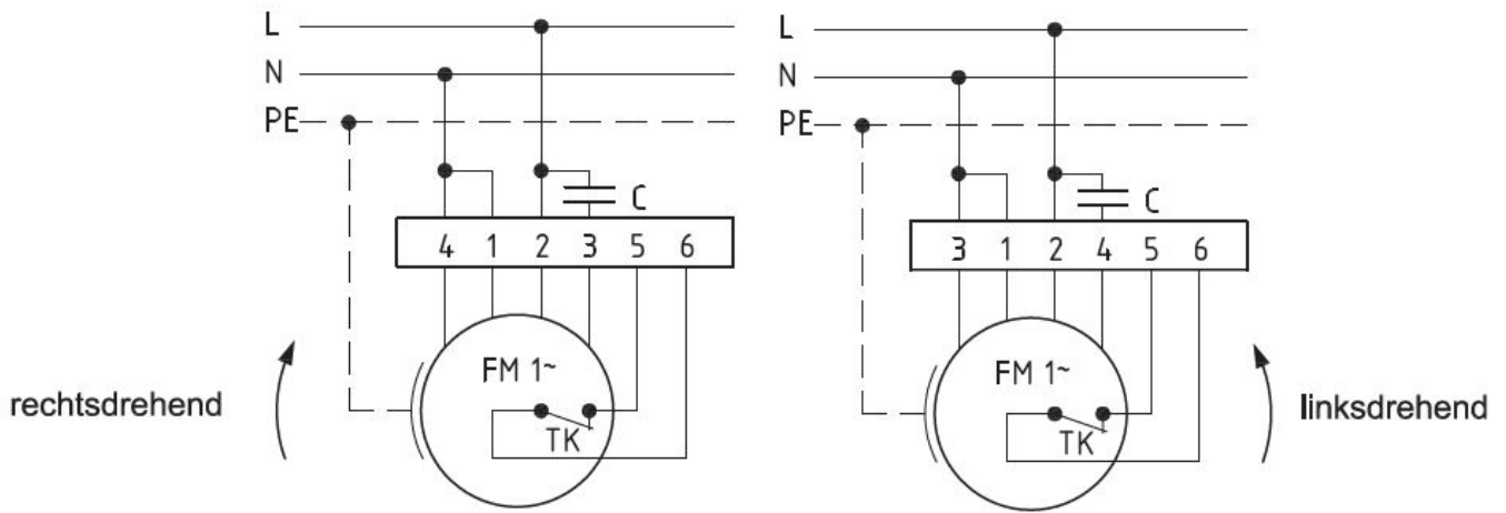
Anschlußplan 0.11-1 r.
