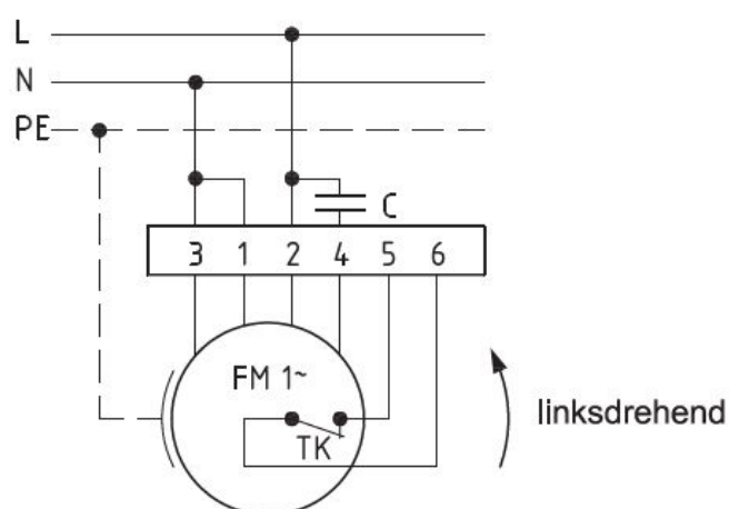
Anschlußplan 0.11-1 l.
