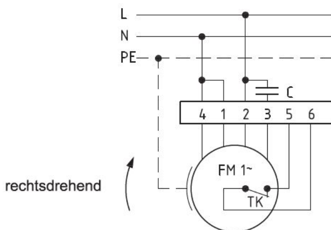
Anschlußplan 0.11-1 r.
