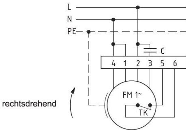
Anschlußplan 0.11-1 r.
