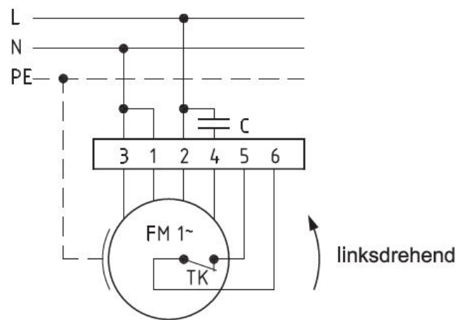
Anschlußplan 0.11-1 l.
