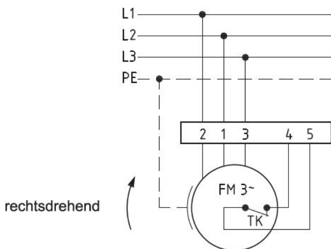
Anschlußplan 0.13-2 r.
